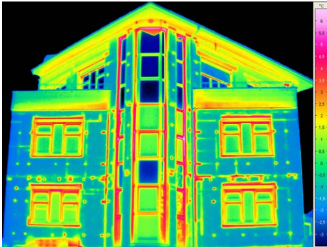
Bild 6: Außenthmografie einer gedämmten Neubaufassade, schlecht verarbeitete Dämmplatten und Dübel als Wärmebrücken erkennbar, unkorrigierte Fenster zeigen den Effekt der Störstrahlung des kalten Himmels
