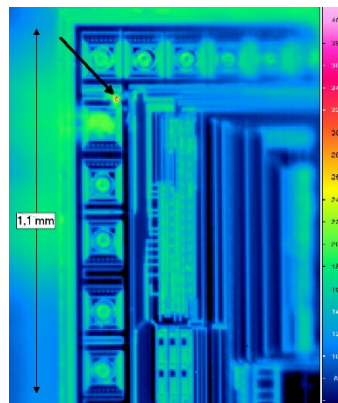
Fehlerhafter Analog-Digital-Wandler mit Leckstrom
