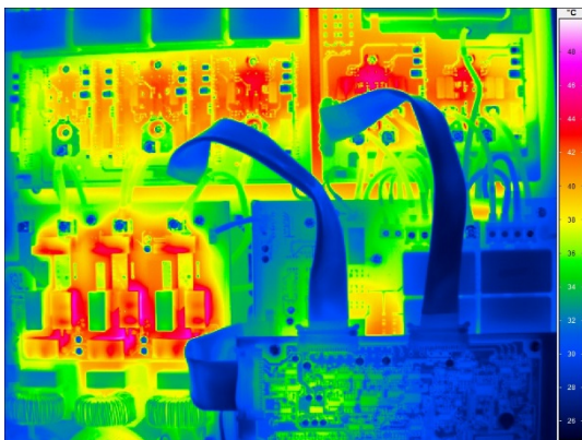
Wechselrichter mit belasteten Bau teilen zur Lebensdauervorhersage
